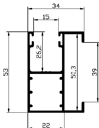
Vodící lišta A8-12 (6-002599-xxxx)
