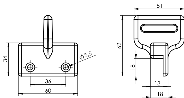
Patka zvýšeného držáku Av – Alu
